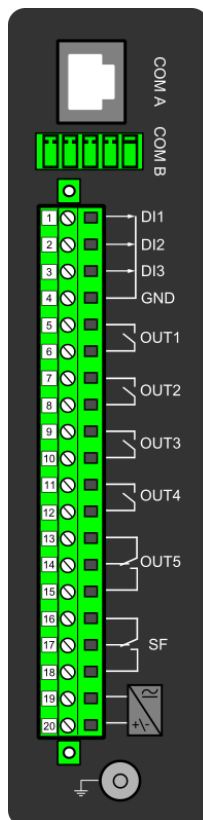
Figure. 8.2 - 211. CPU module.
